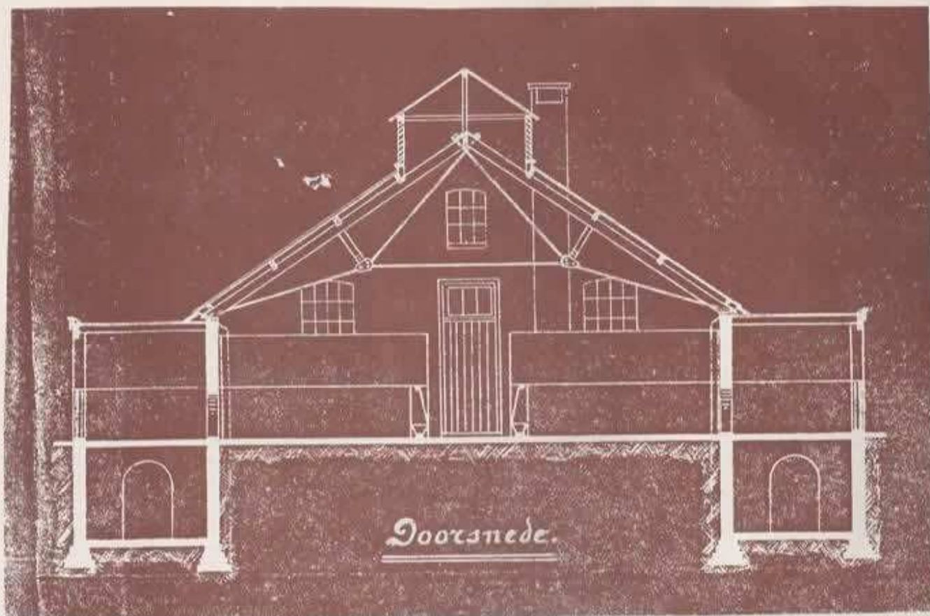
fragment van de bouwtekening uit 1915
